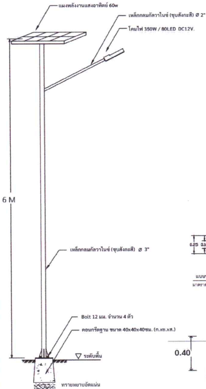
แบบเสาไฟฟ้าพลังงานแสงอาทิตย์ มาตราส่วน 1:25
