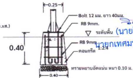
แบบขยายรูปัดฐานราก มาตราส่วน 1:20
