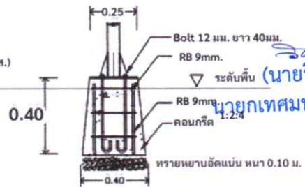
แบบขยายรูปปลั้ฐานราก มาตราส่วน 1:20
