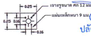
แบบขยายแผ่นเหล็กรับฐานราก มาตราส่วน 1:20
