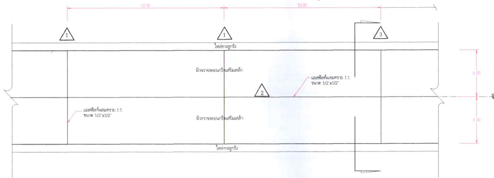
แปลนถนนคอนกรีตเสริมเหล็ก 1:100
