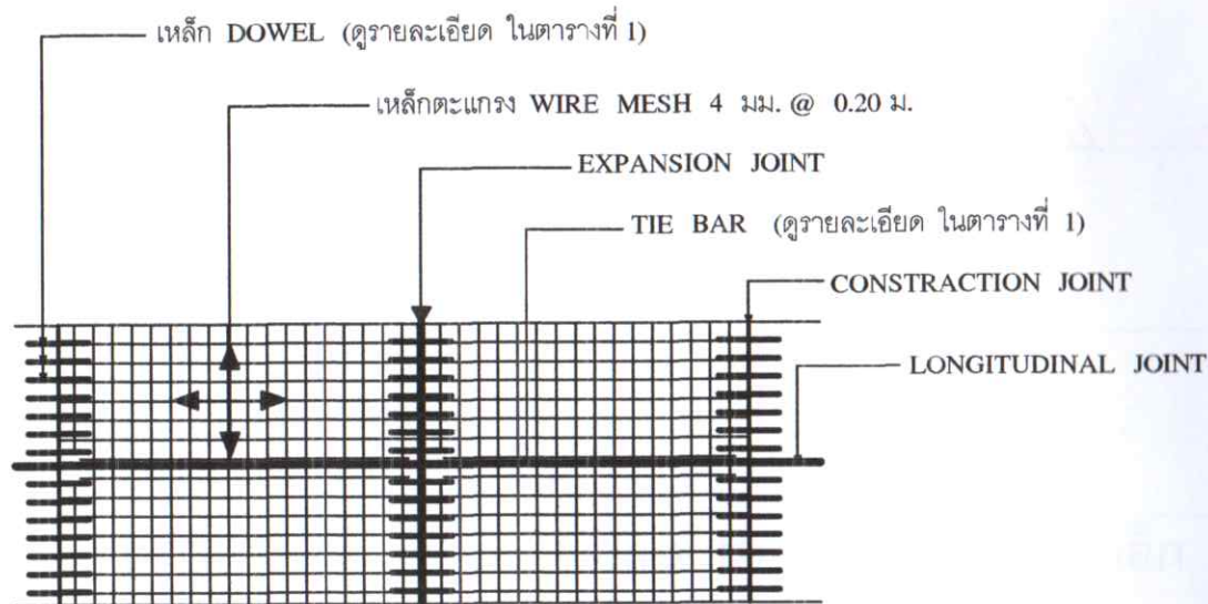
แปลนการวางตระแกรงเหล็ก
