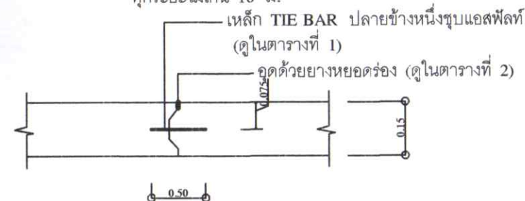
2 LONGITUDINAL JOINT
